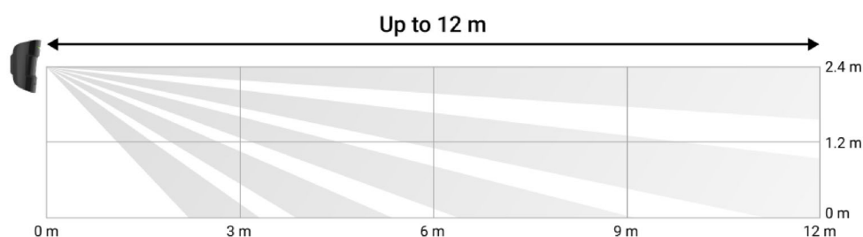
L'angle de vue vertical du détecteur
