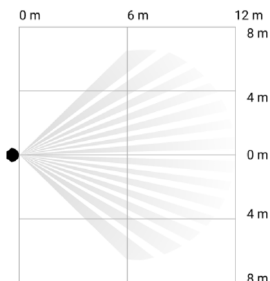
L'angle de vue horizontal du détecteur
